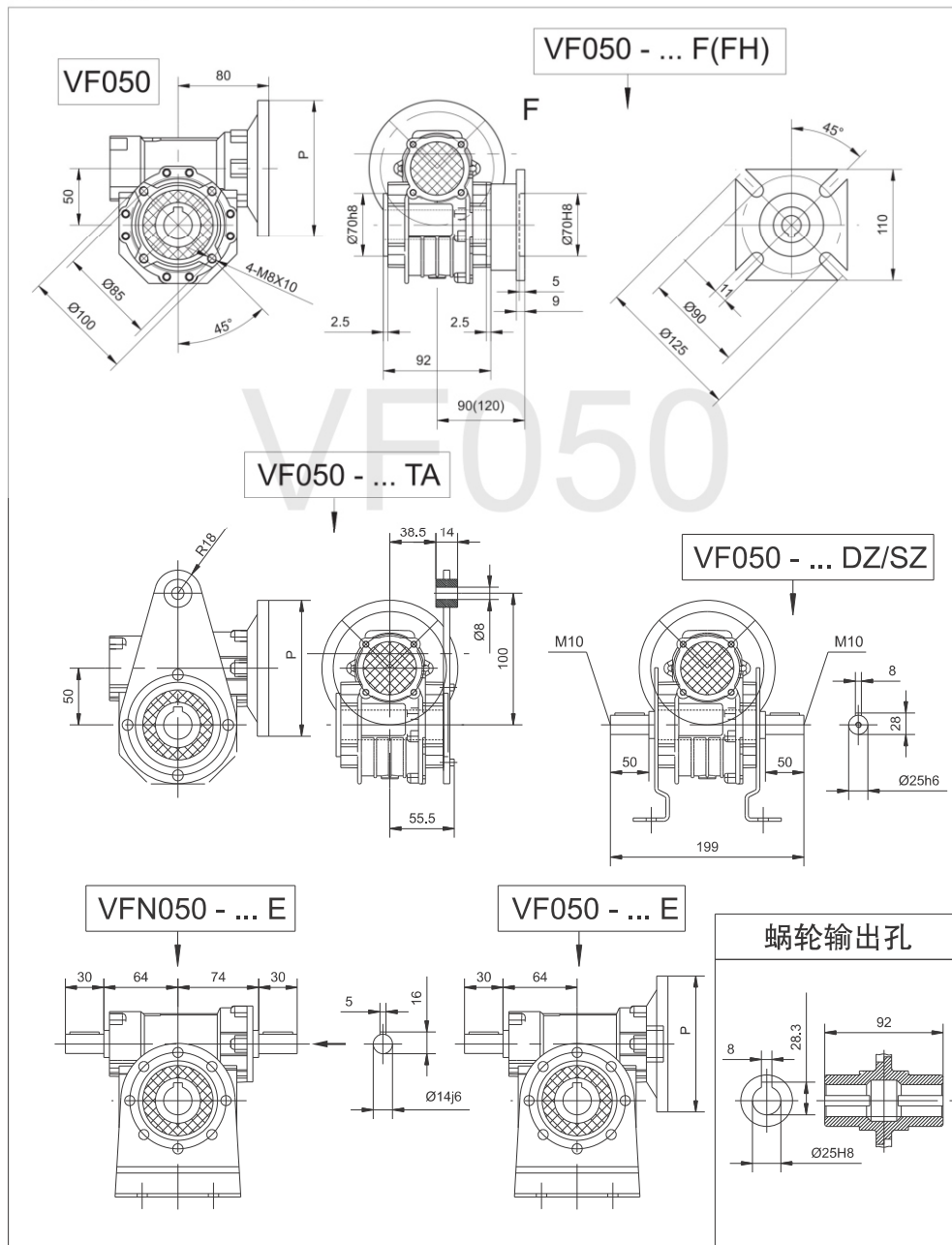
VF050 安装尺寸 P 尺寸见第36页
