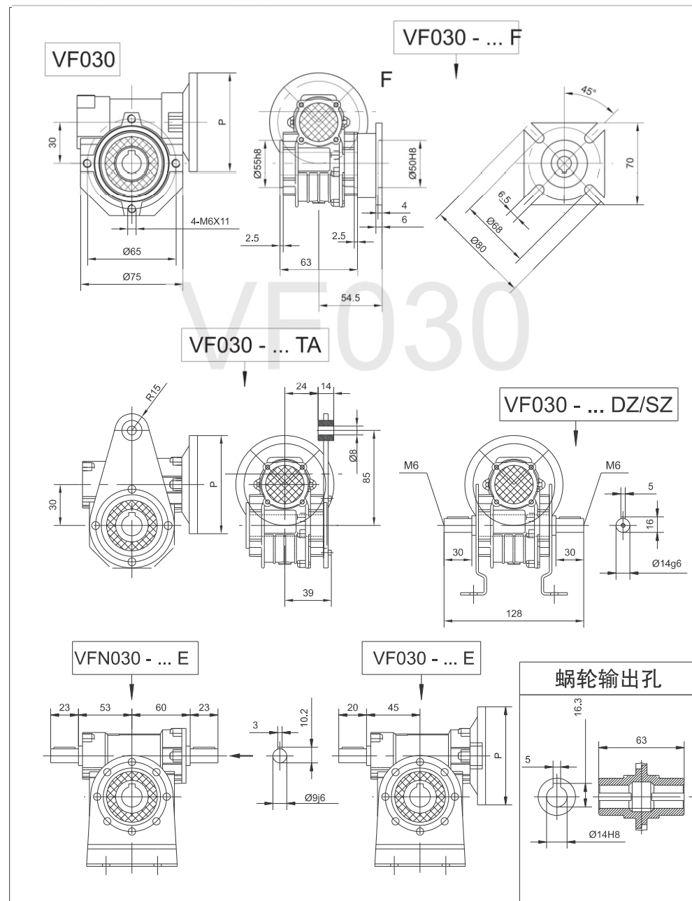
VF030 安装尺寸 P 尺寸见第36页
