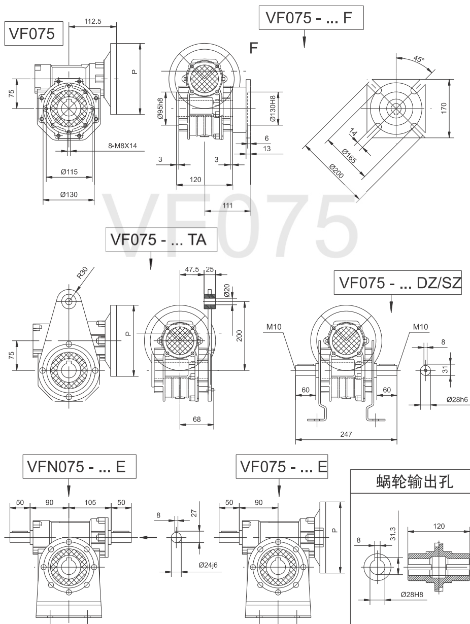
VF075 安装尺寸 P 尺寸见第36页
