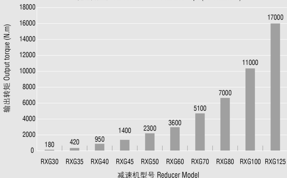
额定转矩表 Selection table of Rated Torque( n_1=900r/min )
